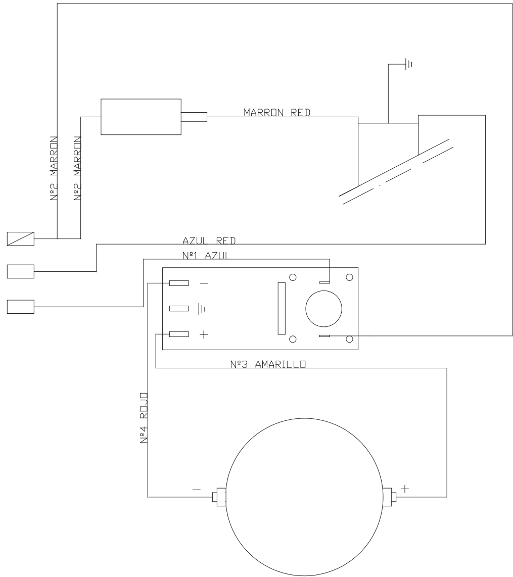
Esquema eléctrico I-1 Timer ■ Electrical Scheme I-1 Timer
